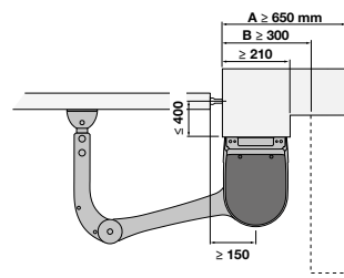
A Braccio intero B Braccio ridotto
